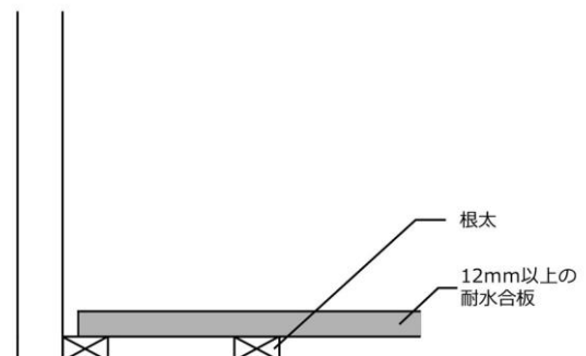
《木組下地の場合》
