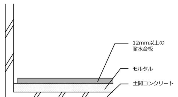
《モルタル直貼りの場合》
